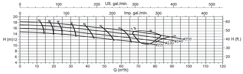
D453-PP 7,5kW
